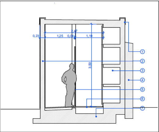
Sezione A-A
