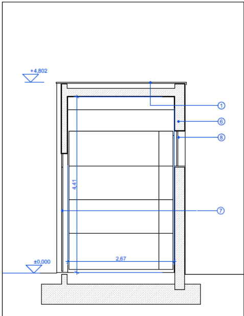
Sezione A-A
