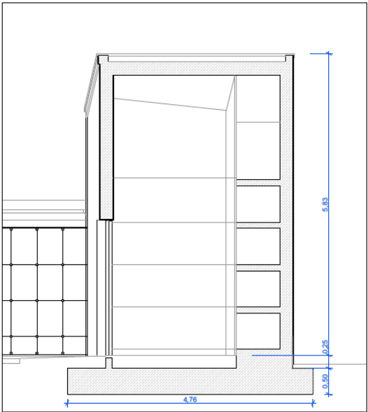
Sezione A-A
