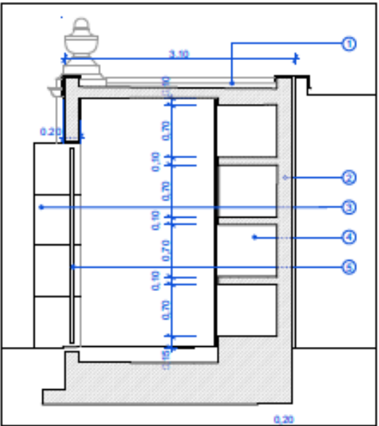
Sezione A-A
